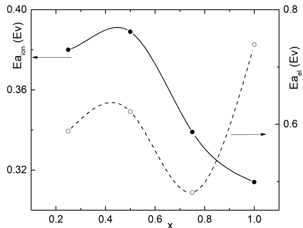
Рис. 4: Концентраційні залежності енергії активації іонної та електронної компонент електричної провідності для керамічних зразків на основі (Cu_{1-x}Ag_x)_7Si_5I .
