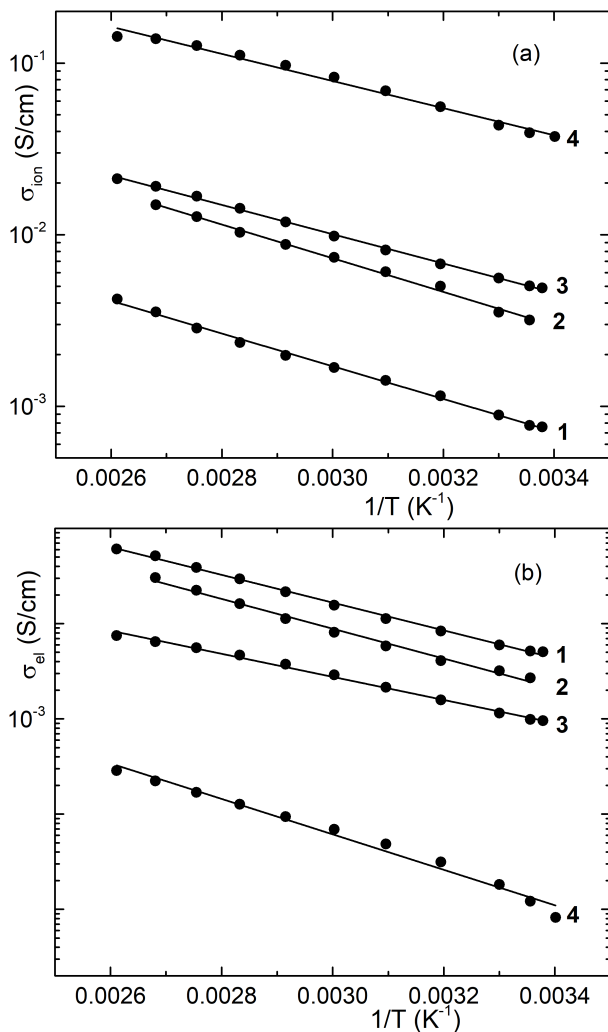
Рис. 3: Температурні залежності іонної (а) та електронної (б) компонент електричної провідності для керамічних зразків на основі (Cu_{1-x}Ag_x)_7Si_5I : (Cu_{0.75}Ag_{0.25})_7Si_5I (1), (Cu_{0.5}Ag_{0.5})_7Si_5I (2), (Cu_{0.25}Ag_{0.75})_7Si_5I (3) та Ag_7Si_5I (4).
