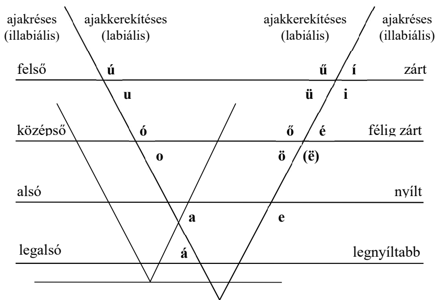
8. ábra. A magyar nyelv magánhangzórendszerének ábrája
