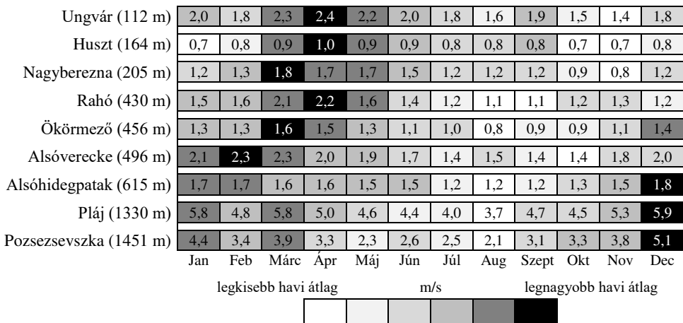
3.2. ábra. A mérőállomások szélességeinek (m/s) havi átlagai 2011–2015 között
