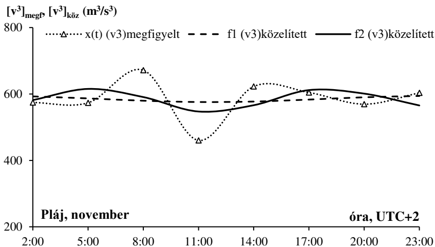
3.29. ábra. A periodikus függvény „legrosszabb” illeszkedése a szélesebbégköbök napi menetére
