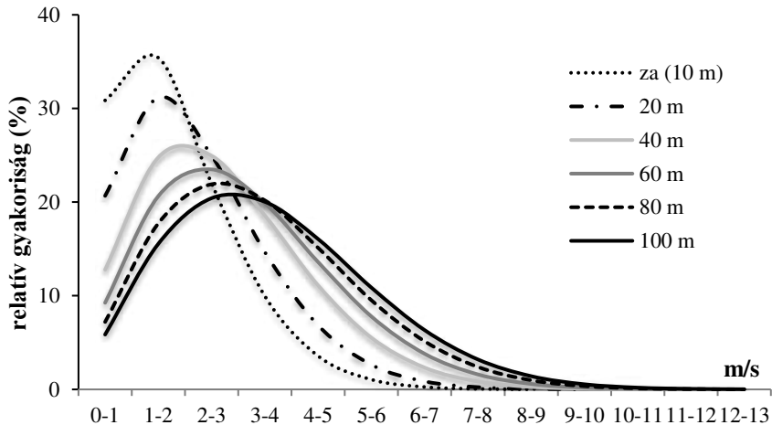
3.16. ábra. A napi átlagos szélesebességek relatív gyakorisági eloszlása Alsóvereckén az anemométer magasságában ( z_a ) és további 5 szinten (2011–2015)
