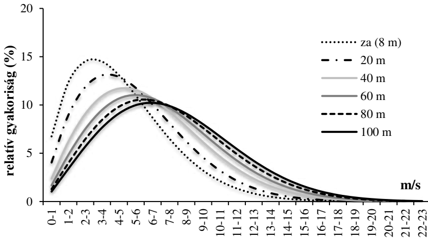
3.17. ábra. A napi átlagos szélsébségek relatív gyakorisági eloszlása a Plájon az anemométer magasságában ( z_a ) és további 5 szinten (2011–2015)
