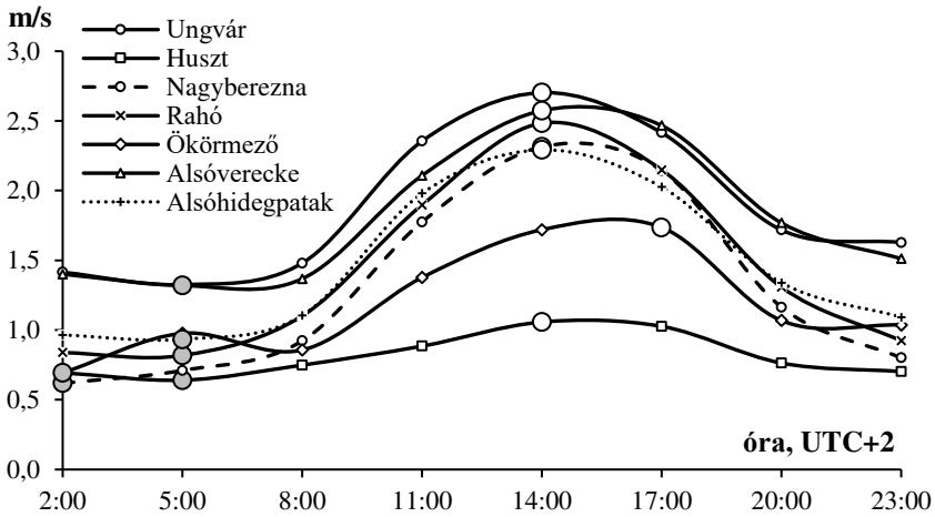
3.7. ábra. Az alföldi és nem alföldi folyóvízgyűjtő állomások terminus időpontokénti átlagos szélességeinek (m/s) napi menete 2011–2015 között (fehér kör jelölő – maximum, szürke kör jelölő – minimum érték)
