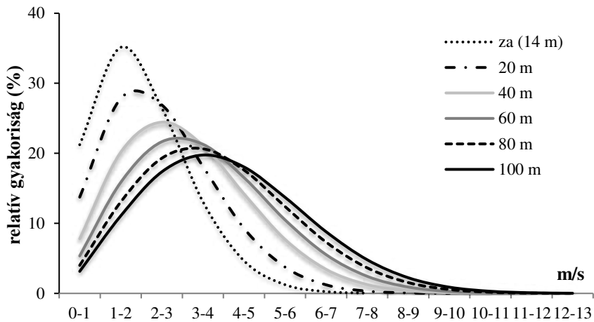
3.15. ábra. A napi átlagos szélesebességek relatív gyakorisági eloszlása Ungváron az anemométer magasságában ( z_a ) és további 5 szinten (2011–2015)
