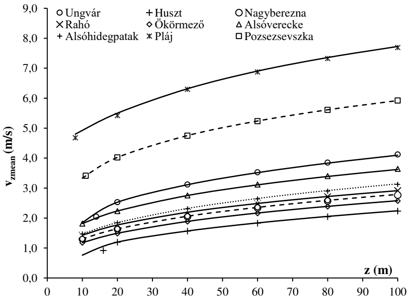
3.18. ábra. Az egész mérési időszakra számított átlagos szélesebbég (pontok) és a rájuk illesztett hatványfüggvény (vonalak)
