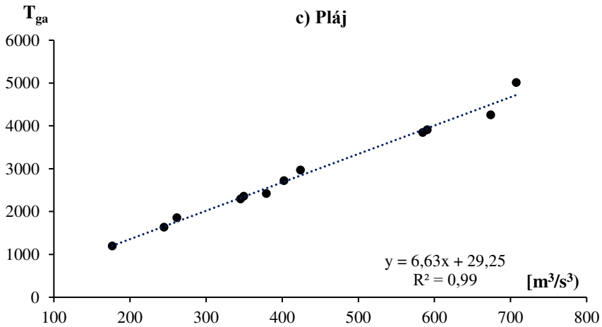
3.34. ábra. A havi átlagos fajlagos széltejesítménnyel arányos görbe alatti terület ( T_{ga} ) és a szélesebbesség köbök havi átlaga ( v_m ) közötti lineáris korreláció és regresszió a) Ungvár, b) Rahó és c) Pláj állomás esetében (10 m magasságban)
