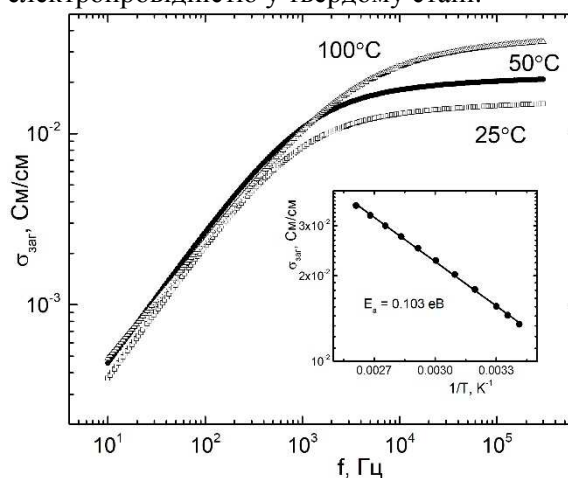
Рис. 4. Частотна залежність загальної електропровідності для керамік виготовлених на основі мікрочасталічних порошоків твердих розчинів \text{Ag}_{6+x}(\text{P}_{1-x}\text{Ge}_x)\text{S}_5\text{I} на прикладі \text{Ag}_{6.25}(\text{P}_{0.75}\text{Ge}_{0.25})\text{S}_5\text{I} .
